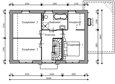
1ste Verdieping
