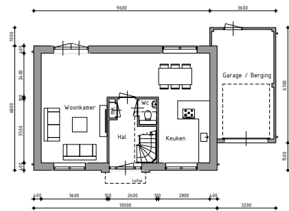
Begane grond
