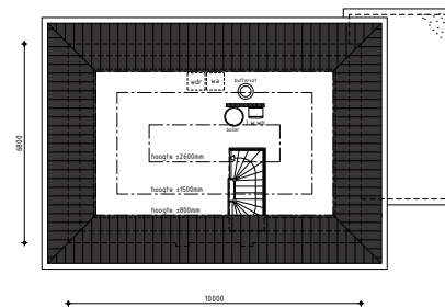
2de Verdieping
