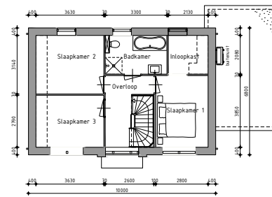
1ste Verdieping
