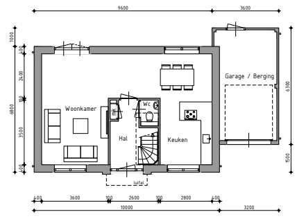
Begane grond
