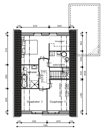
1ste Verdieping
