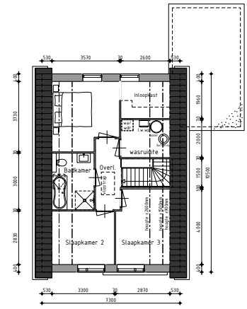
1ste Verdieping
