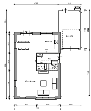
Begane grond
